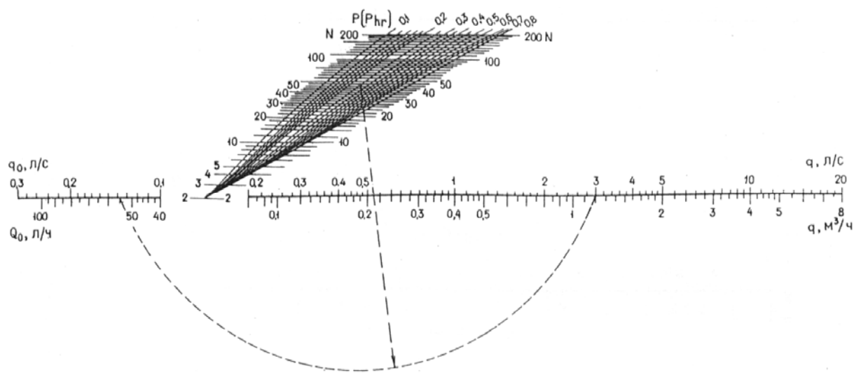
Черт. 3. Номограмма для определения секундных и часовых расходов воды q при q(0) \leq 0,3 \text{ л/с} , N \leq 200 и P > 0,1
